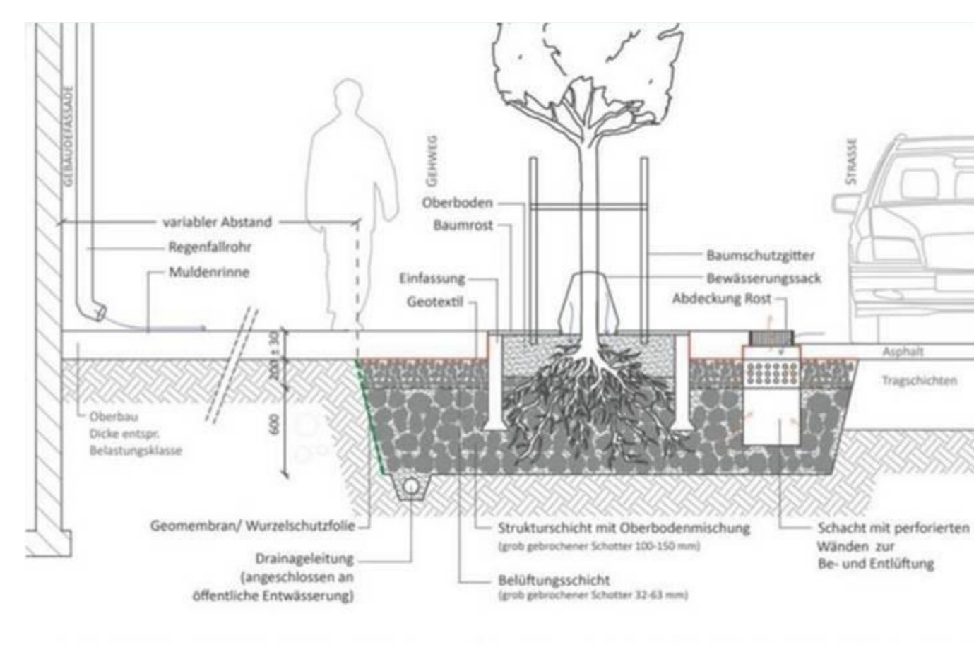
System Stockholm: Einleitung von Straßenabflüssen in die Pflanzgrube gemäß der Stockholm Solution (siehe Maßstab), Grafik: C.Bibber.
